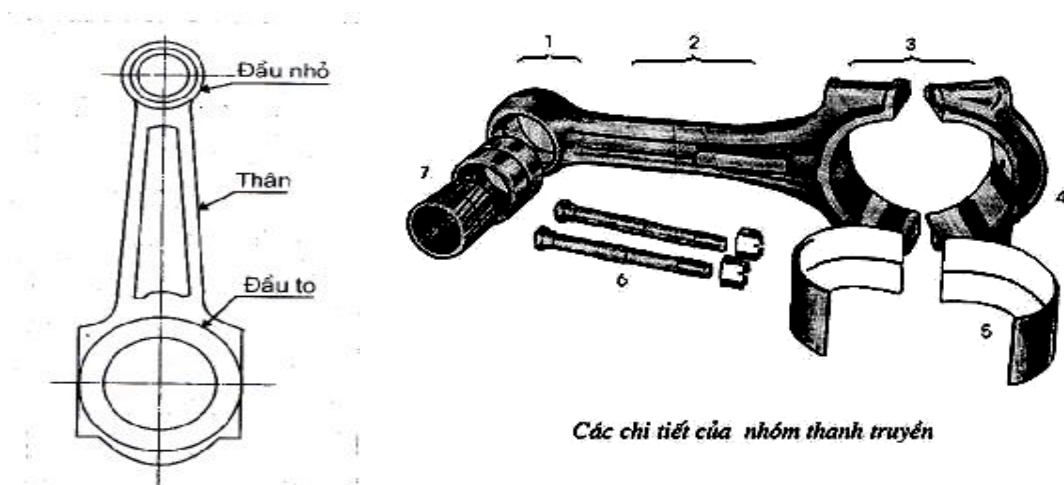
Hình 1.12. Thanh truyền.
