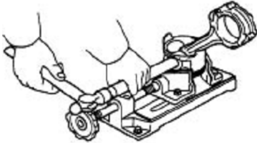
Hình 5.9 Đồ gá tiện piston vòng gang.
