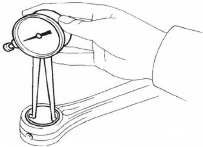
Hình 6.1 Kiểm tra lỗ dầu nhỏ thanh truyền.
