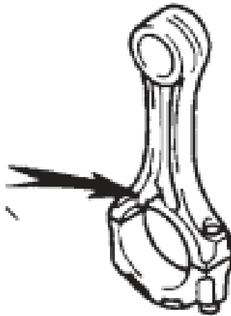
Hình 6.2 Kiểm tra lỗ dầu to thanh truyền.
