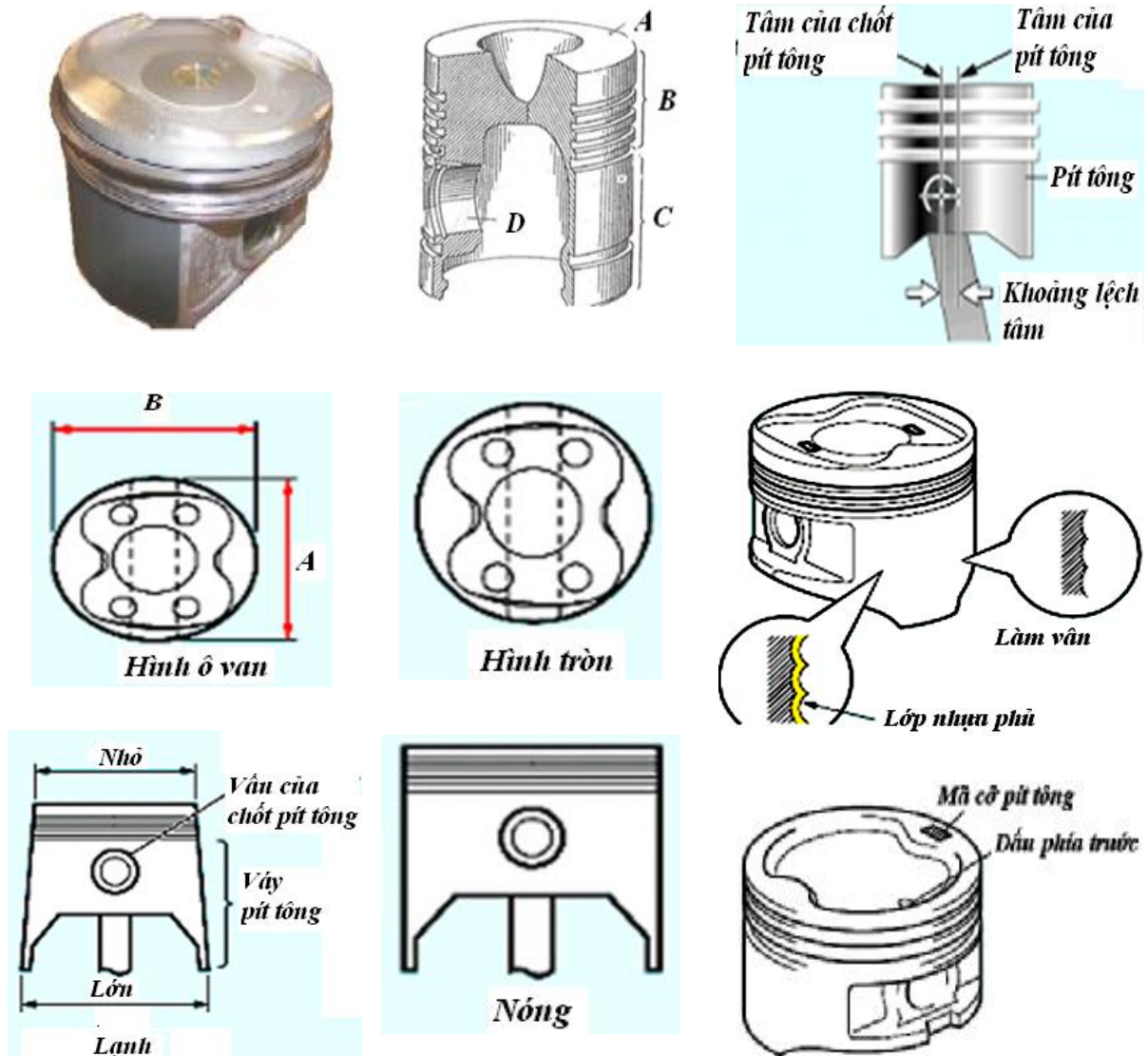
Hình 1.6 Piston.
