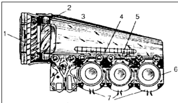
Hình 4.4. Hệ thống làm mát bằng không khí
