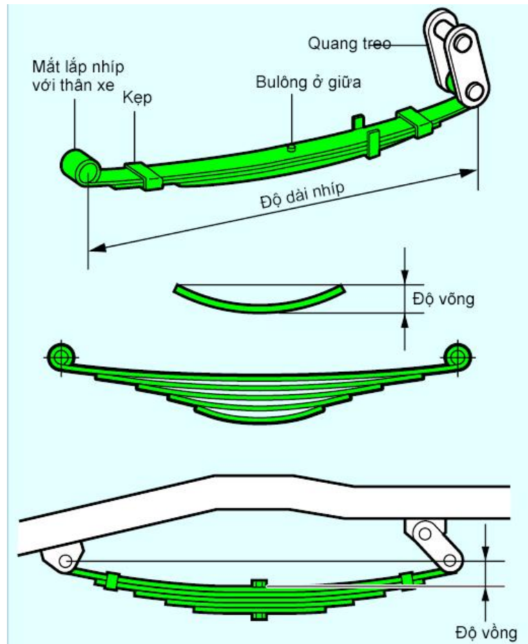
Hình 1.18. Nhíp lá
